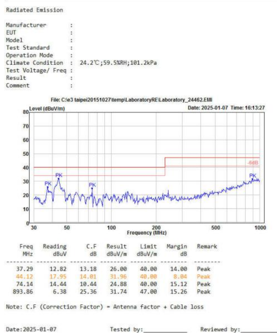
图 5-7 辐射测试垂直方向
