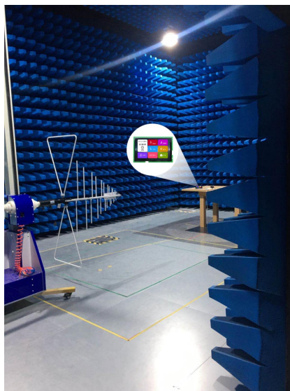
图 5-5 辐射测试图
